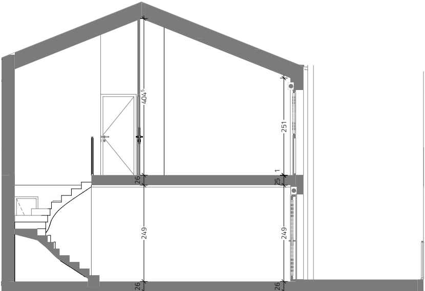
COUPE AA
